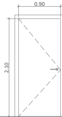
P-04 (0.90 x 2.10 m) 2 u Porta metàl·lica batent, amb pany i clau de seguretat. Porta de manteniment. Espais sense us ni ocupació. EI60
