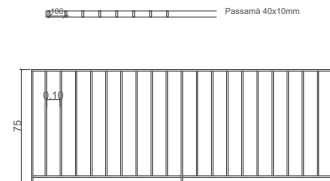
B-04 1u - 16.00 ml Barana amb passamà superior i inferior de 40 x 10 mm, i barrots de 40 x 10 mm. Pintura amb dos imprimacions anti-oxid i 2 mans d'acabat oxidon "gris - negra).
