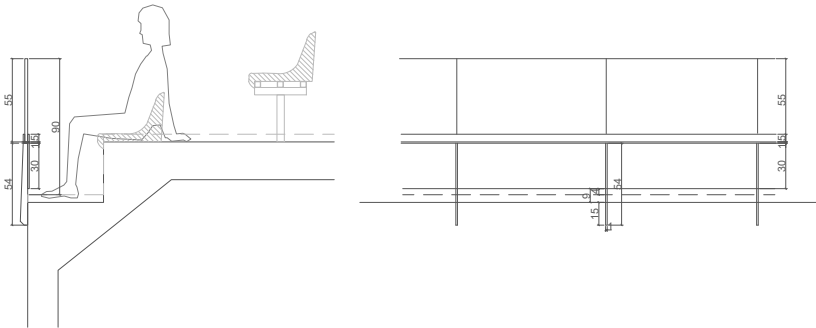
B-01 1u - 45.50 ml Barana de vidre laminat de seguretat 20,8mm subjectat a base de peus amb platina amb pinça incorporada. Part metàl·lica pintada Ral 7016 Segons CTE DB SE-AE - Zona C2 - Força horitzontal 0,8 KN/m. UNE 85238:1991
