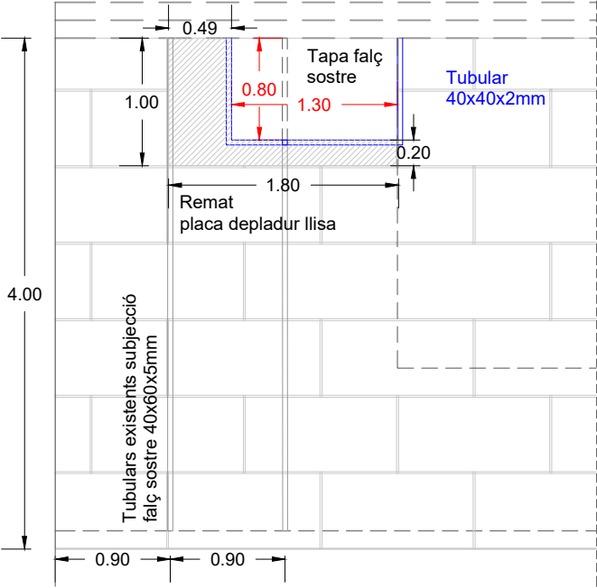
Nivell falç sostre Subjecció tapa de registre
