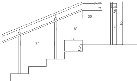
B-02 1u - 3.00 ml / 1u - 4.50 ml / 1u - 5.00 ml Barana escala espai públic est. Passama superior diam 40mm i inferior 30mm, anclat al terra. Pintura amb dos imprimacions anti-oxid i 2 mans d'acabat oxidon "gris - negra).
