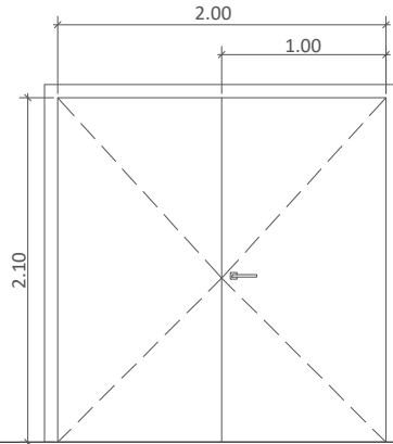
P-03 (2.00 x 2.10 m) 1 u Porta de doble batent EI60 amb detector de bloqueig Pintat Ral 7016
