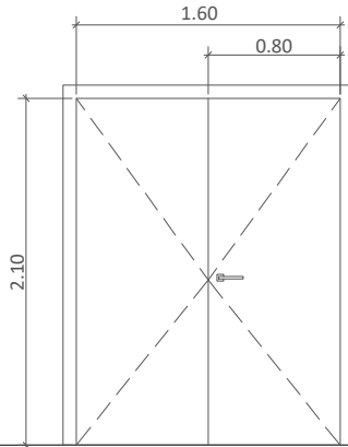
P-02 (1.60 x 2.10 m) 1 u Porta de doble batent amb pany i clau. Pintat exterior Ral 7016 i interior groc existent
