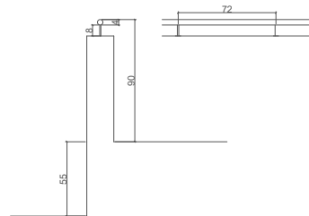
B-03 1u - 14.50 ml Paret de formigó de 20cm de gruix amb passamà superior de diam 40mm, anclat al mur. Pintura amb dos imprimacions anti-oxid i 2 mans d'acabat oxidon "gris - negra).
