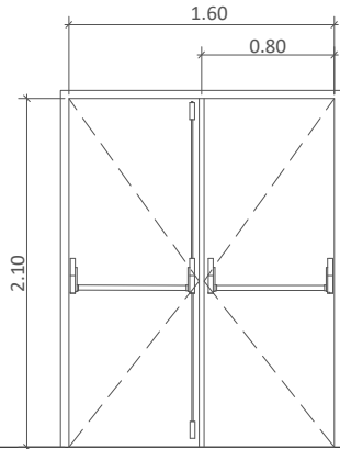
P-01 (1.60 x 2.10 m) 2 u Porta d'emergència doble batent amb barra horitzontal d'empenta. Pintat exterior Ral 7016 i interior groc existent
