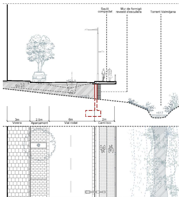
Figura 77: Secció de la ronda de Montserrat on es contempla la instal·lació del carril bici en paral·lel al pas del Torrent Valmitjana.
