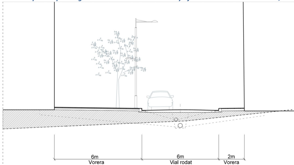
Figura 68: Secció tipus del perllongament de la carretera de Balenyà fins a la ronda de Montserrat, de 14 metres.
