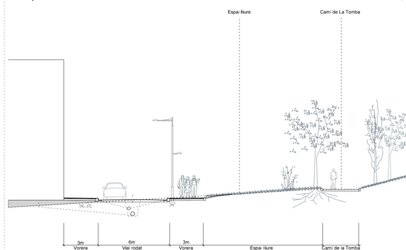
Figura 66: Secció tipus del nou vial de connexió entre el carrer de Vic i la ronda de Montserrat, de 10 metres.
