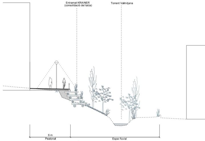
Figura 67: Secció tipus del nou vial de connexió entre el carrer de Vilanova i la ronda de Montserrat, de 6 metres.
