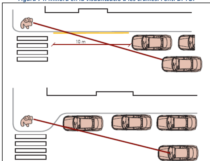
Figura 74: Millora en la visualització a les cruïlles. Font: DPTOP
