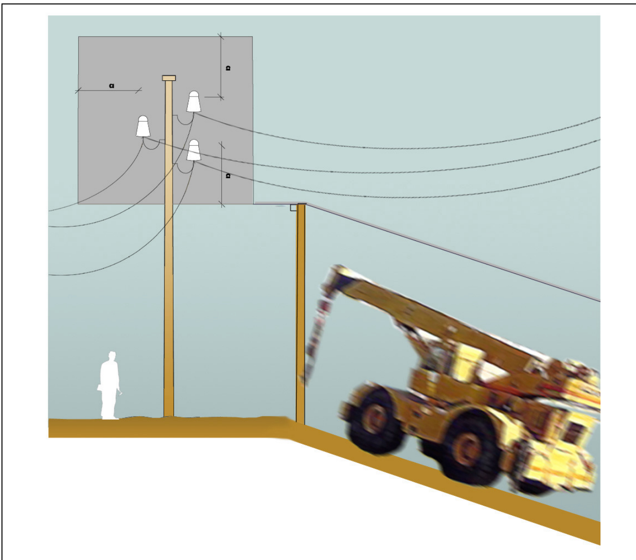
Esquema de pas per sota de línies aèries de Baixa Tensión a=2.00\text{m} .
