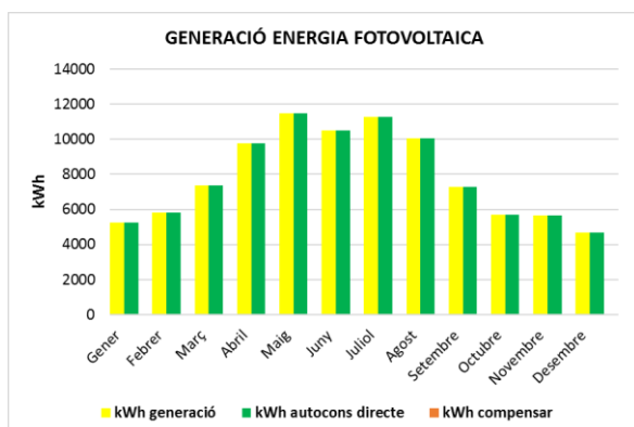
Figura 13 Generació fotovoltaica
