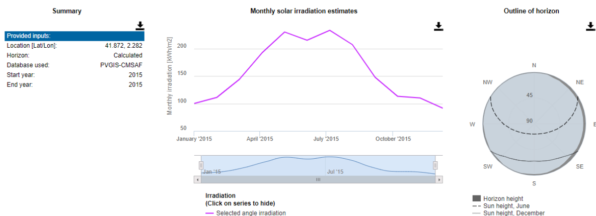
Figura 11 Dades de radiació obtingudes de PVGIS [kWh/m 2 ]
