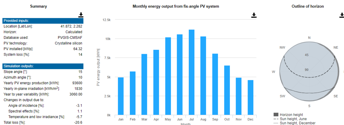
Figura 12 Producció solar estimada.
